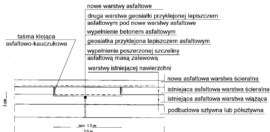
Rys. 3. Naprawa głęboko pojedynczego pęknięcia odbitego, w przypadku braku dobrego podparcia krawędzi pęknięcia
